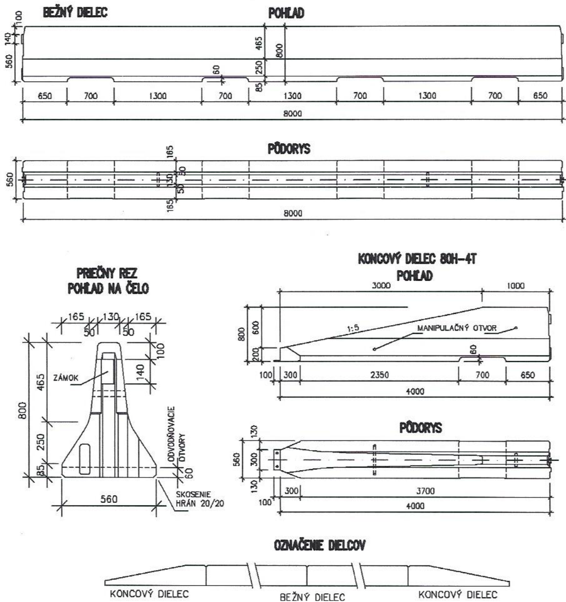
Obrázok 3 – Obojstranné betónové zvodidlo RB 80H-8, bežný a koncový dielec, v [mm]
