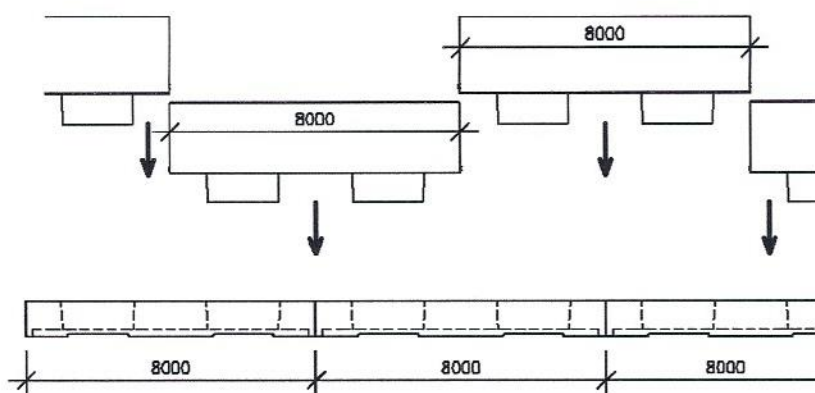
Obrázok 17 – NB 100/300-8, schéma montáže, v [mm]
