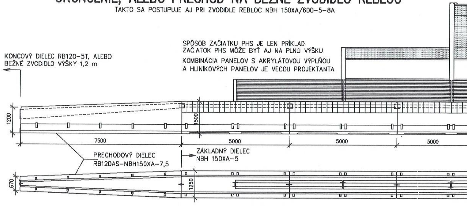
Obrázok 24 – NBH 150XA/600-5, ukončenie alebo prechod na betónové zvodidlo, v [mm]
