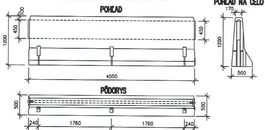
Obrázok 33 – Rozvetvenie zvodidla RB 120.1-7,5 v [mm]
