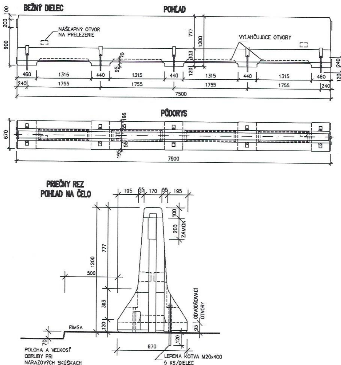
Obrázok 15 – Betónové zvodidlo RB120A-7,5, v [mm]
