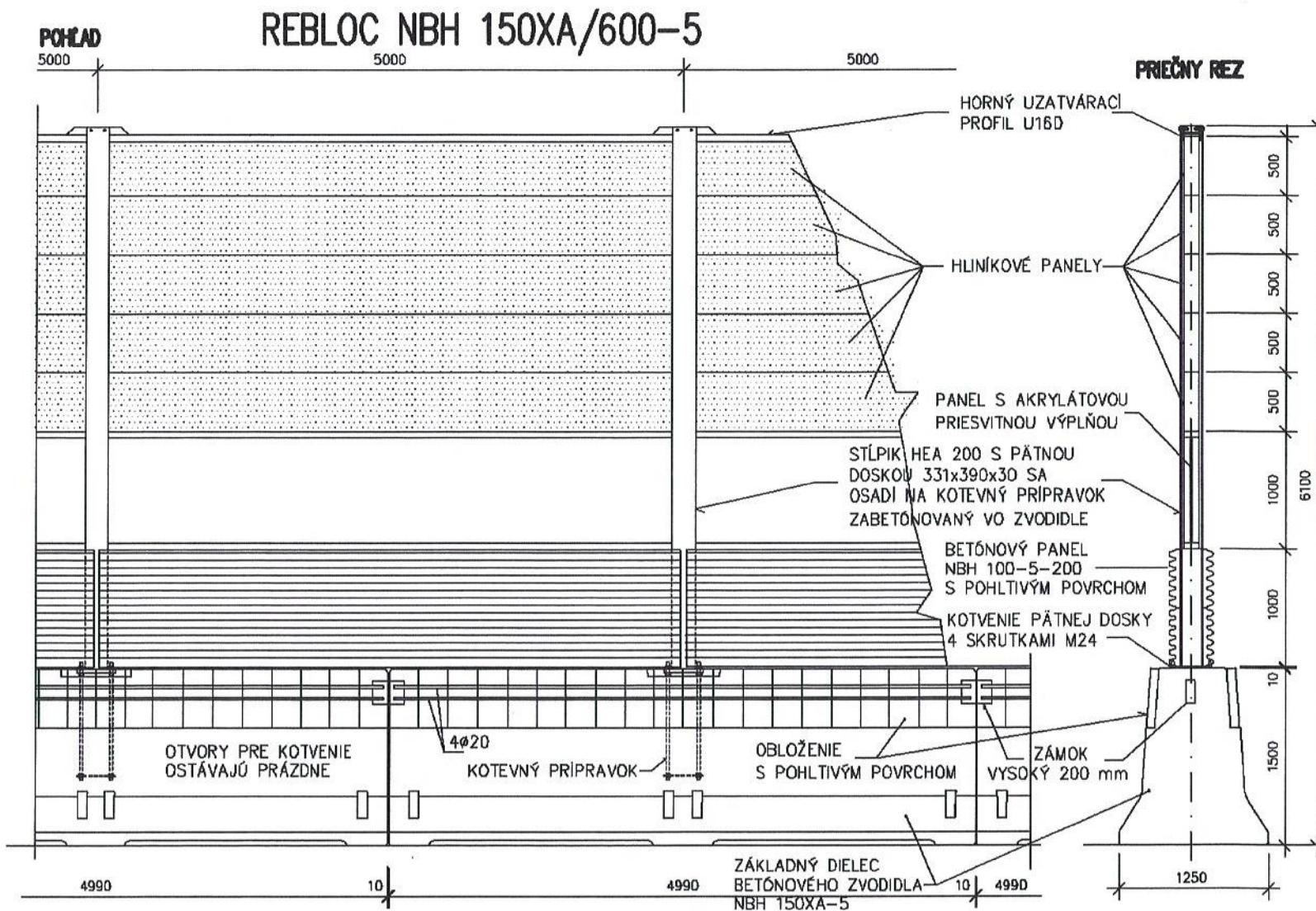
Obrázok 23 – NBH 150XA/600-5, v [mm]
