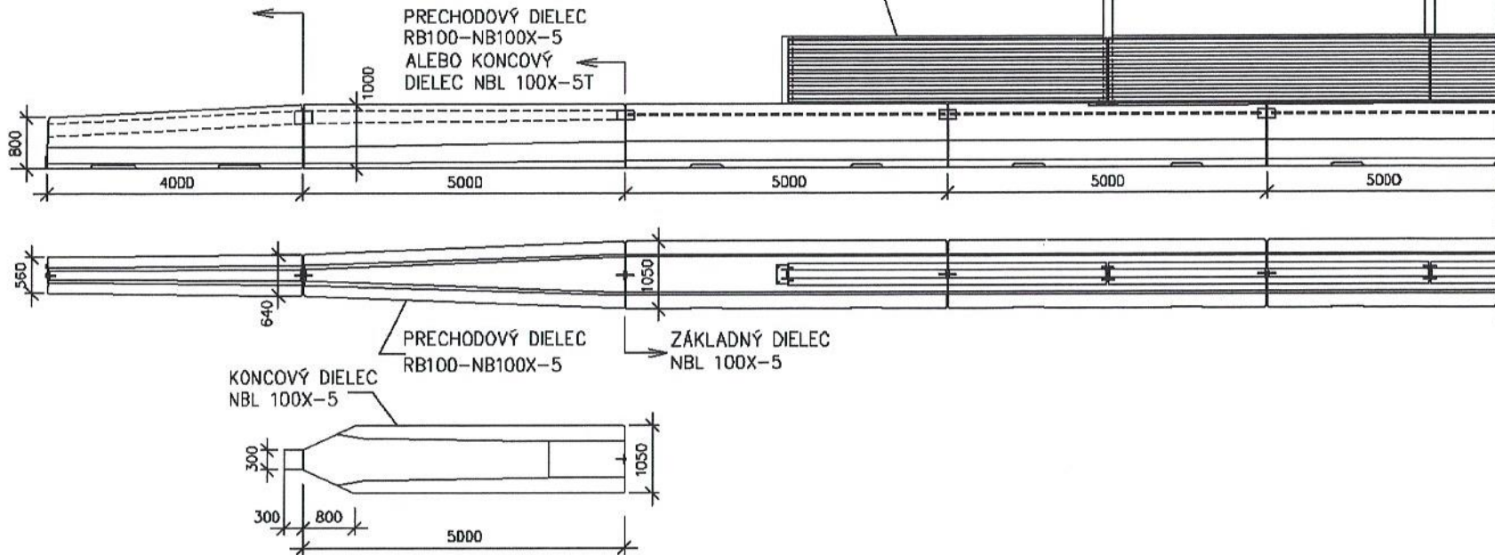
Obrázok 21 – NBL 100X/400-5, ukončenie alebo prechod na betónové zvodidlo, v [mm]
