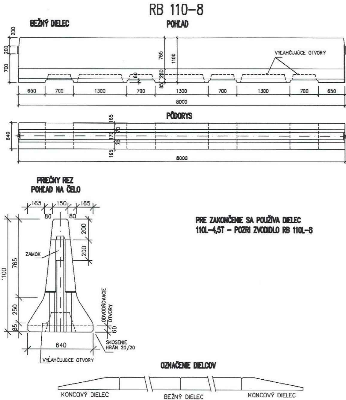
Obrázok 9 – Obojstranné betónové zvodidlo RB 110-8, bežný a koncový dielec, v [mm]
