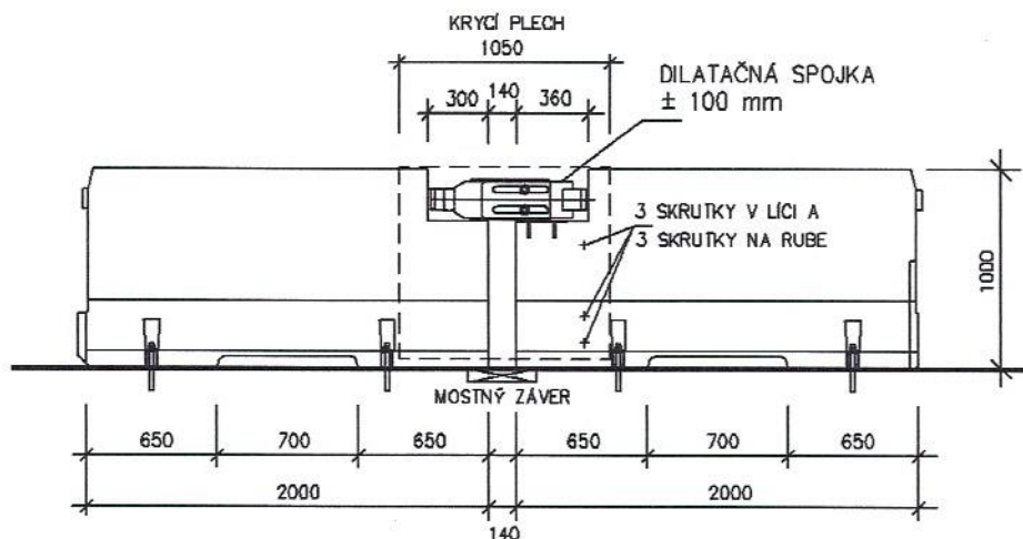
Obrázok 27 – Dilatácia zvodidla RB 100A-8, v [mm]
