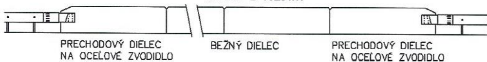
Obrázok 30 – Prechod na ocelové zvodidlo, v [mm]
