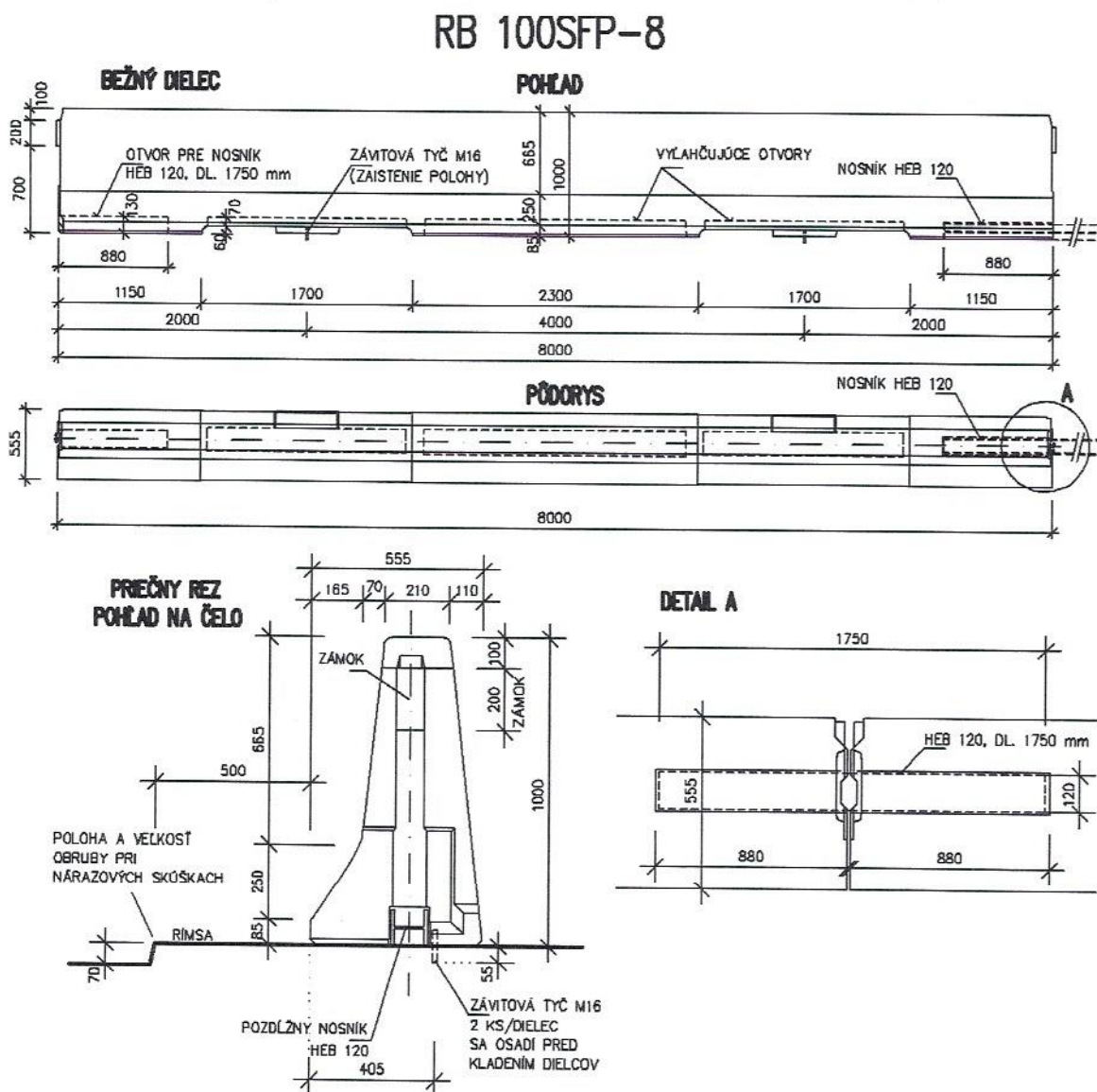
Obrázok 13 –Betónové zvodidlo RB 100SFP-8, v [mm]
