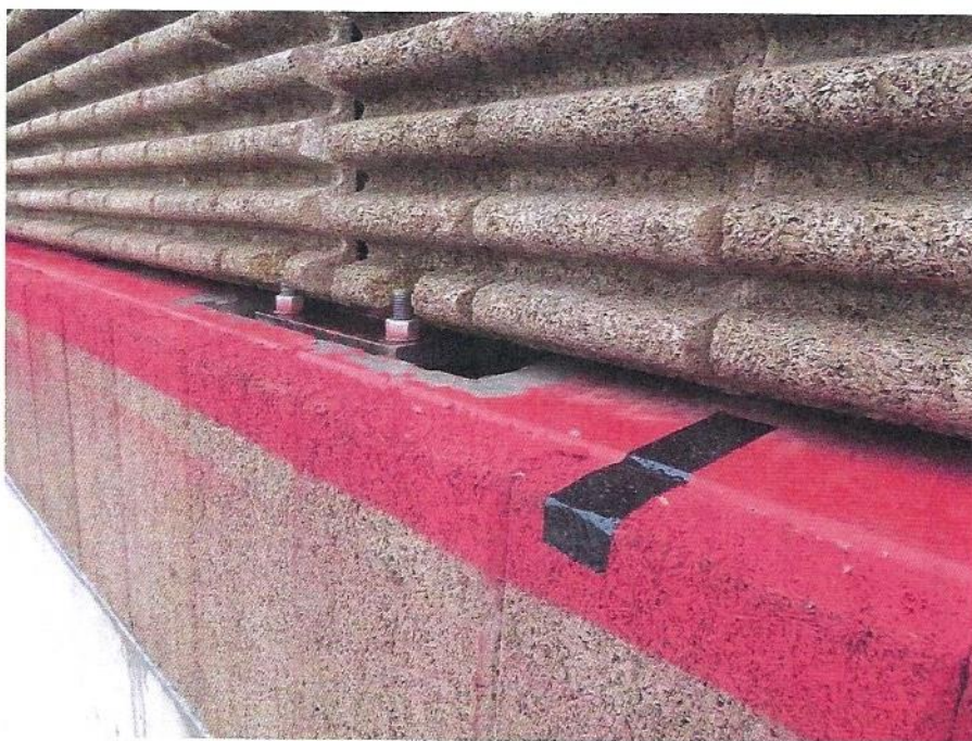
Obrázok 22 – Betónové zvodidlo NBH 150XA/600-5 detail protihlukových materiálov
