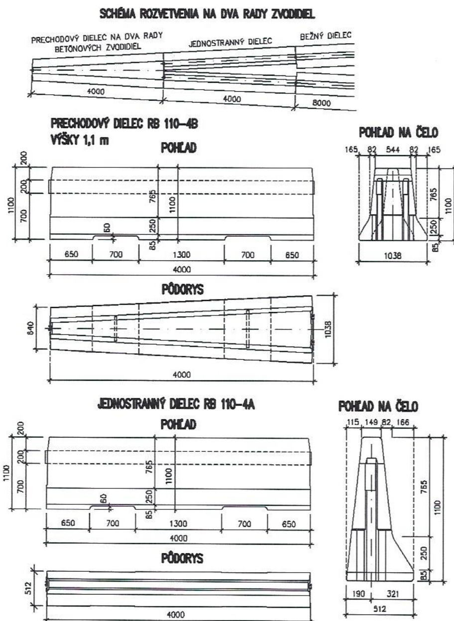
Obrázok 32 – Rozvetvenie zvodidla RB 110-8, v [mm]
